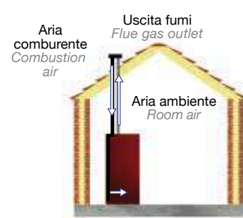
3. Funzionamento con aria comburente preriscaldata prelevata dall'ambiente esterno attraverso il tubo coassiale, in modo indipendente dalla stanza di installazione. Operation with preheated combustion air drawn from outdoors through the concentric pipe and not from the room of installation.
