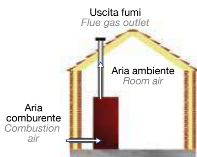
2. Funzionamento con aria comburente prelevata dall'ambiente esterno in modo indipendente dalla stanza di installazione. Operation with combustion air drawn from outdoors and not from the room of installation.
